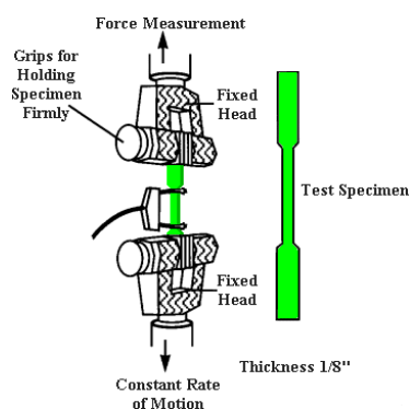
Fig 8 Tensile Strength
